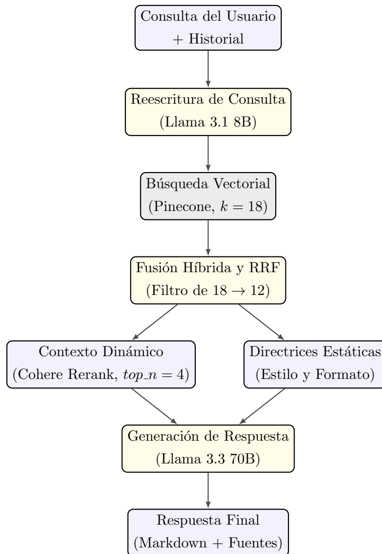
Figura 6.4: Flujo de datos y arquitectura del sistema Dual RAG
